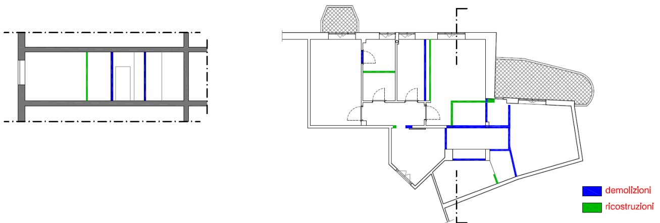
demolizioni / ricostruzioni sc.1:100
